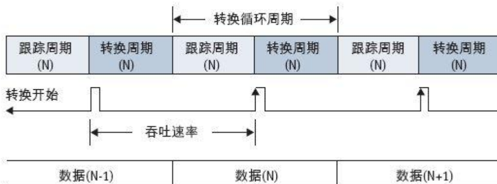
图1：ADC转换循环。
