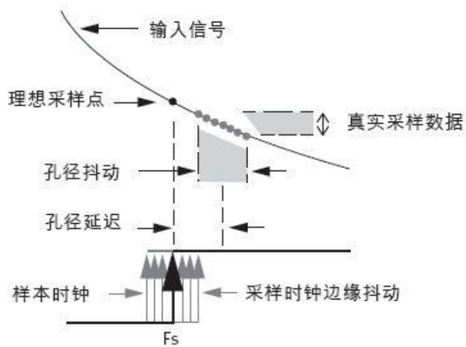
图2：孔径抖动和延迟。
